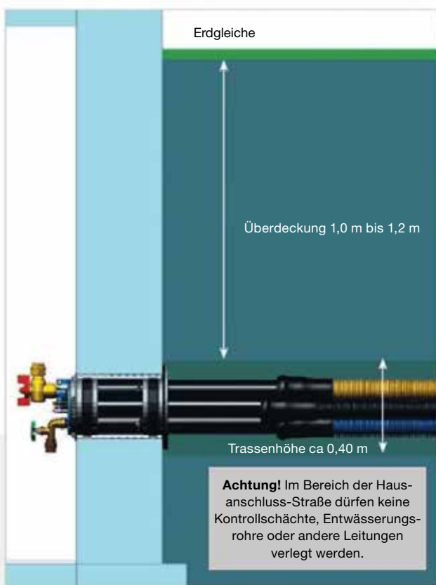
Seitenansicht
