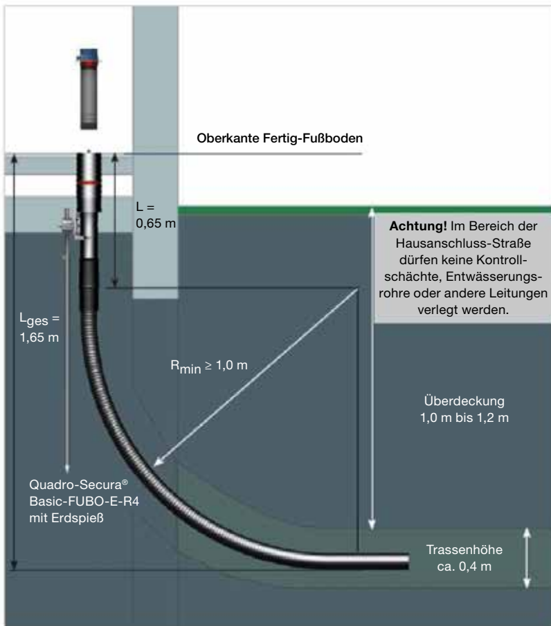
Seitenansicht
