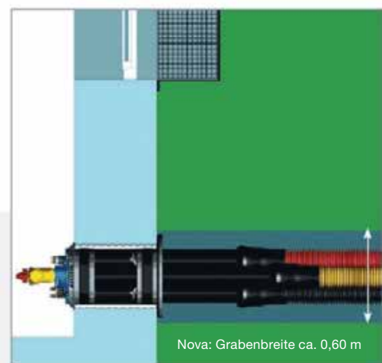
Draufsicht
